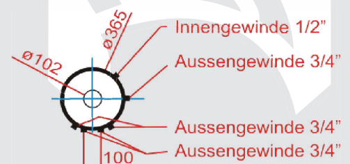
Anschlüsse ZW100
